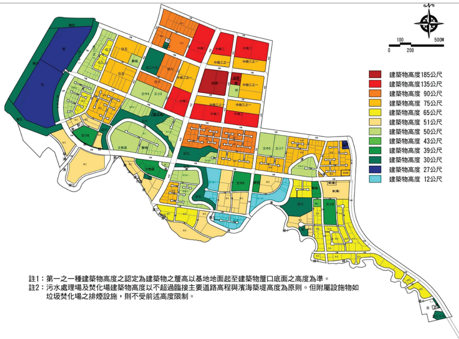
附圖六 各街廓建築物高度管制規定示意圖
