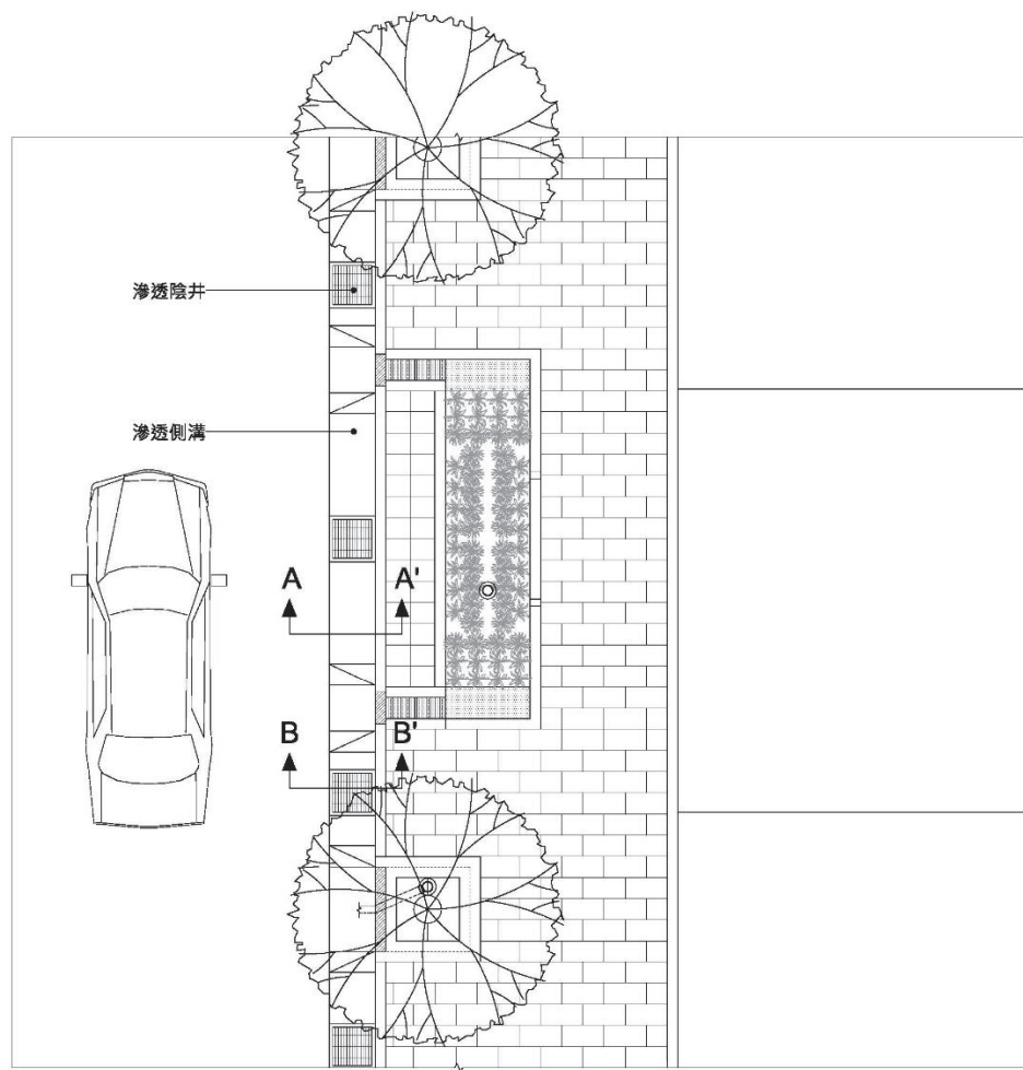
附圖十七 滲透陰井及滲透側溝示意圖說
