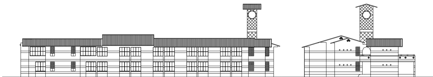
南向立面圖
