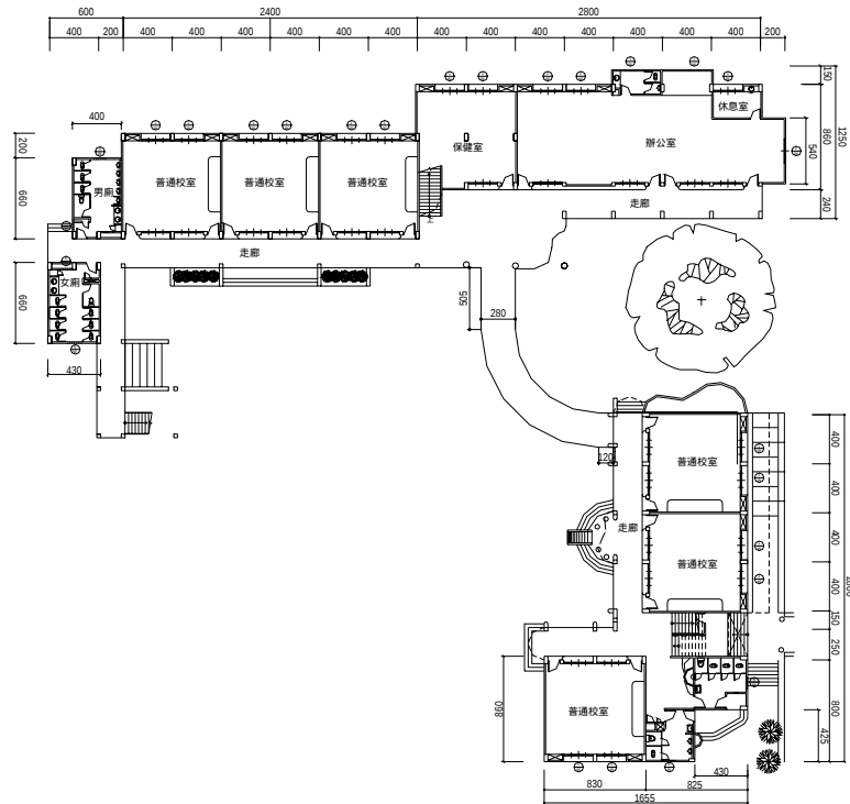
一層平面圖
