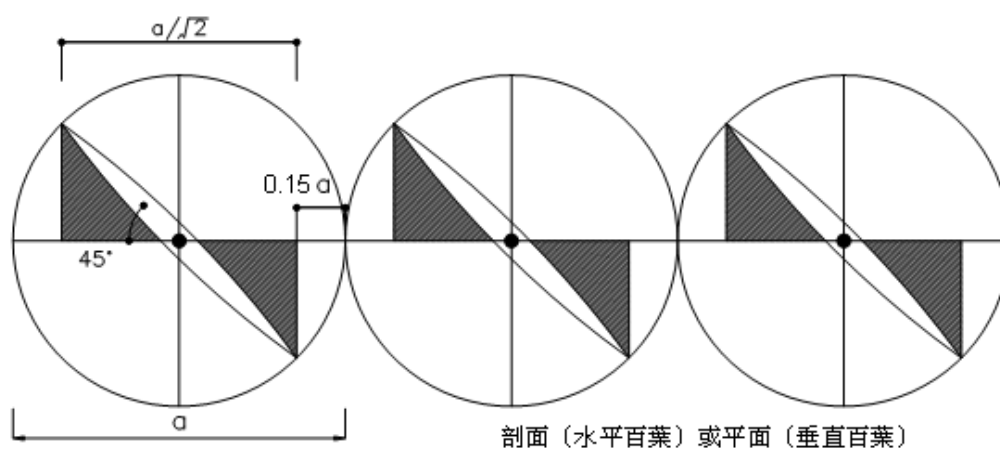
圖 8 自動百葉遮陽之 K_i 模擬值
