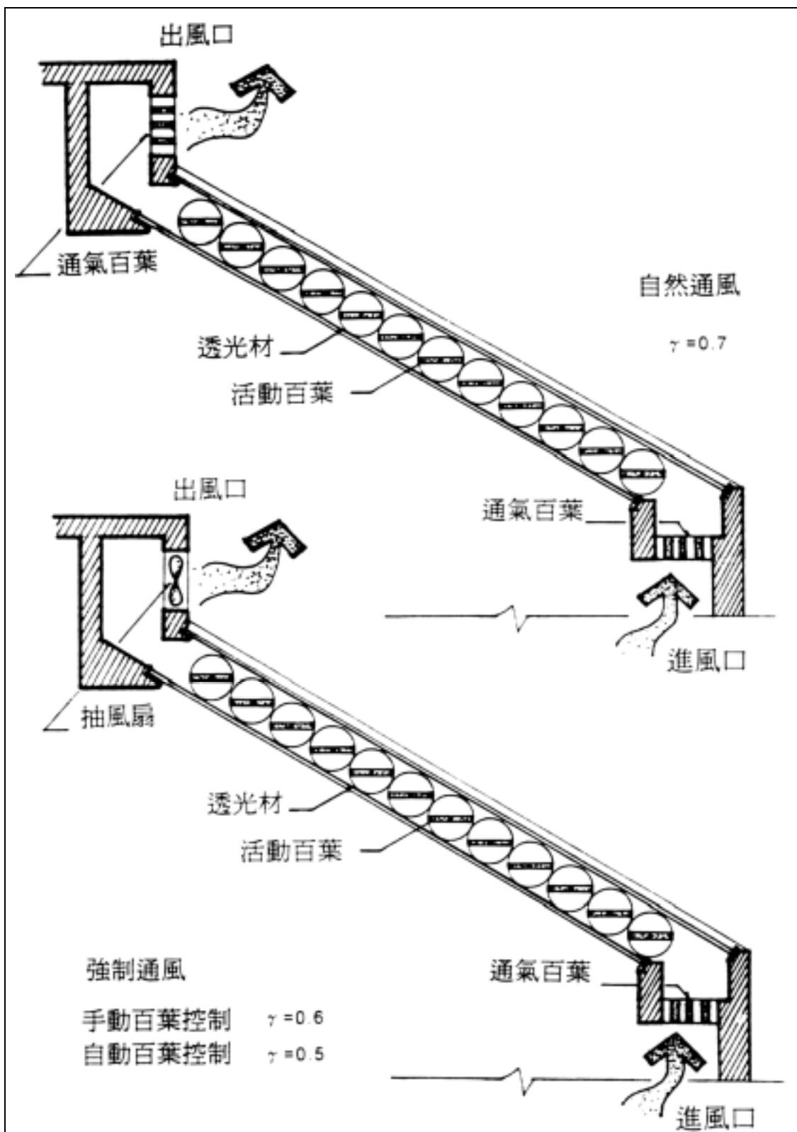
圖 3 雙層氣流窗空氣層內含百葉之圖例
