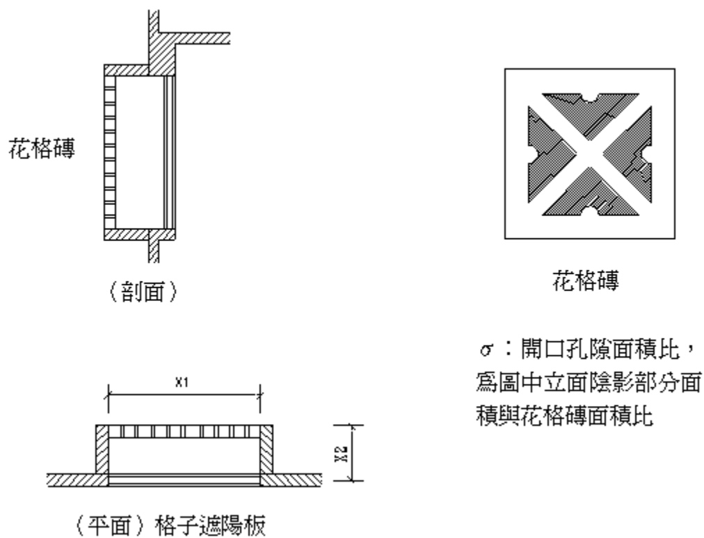
圖 7 花格磚或類似之遮陽裝置，其 K_i 值應以其開口孔隙面積比 \sigma 乘上形狀接近之格子遮陽之 K_i 值，即 K_i = (\sigma \times \text{形狀相近格子遮陽之 } K_i \text{ 值})
