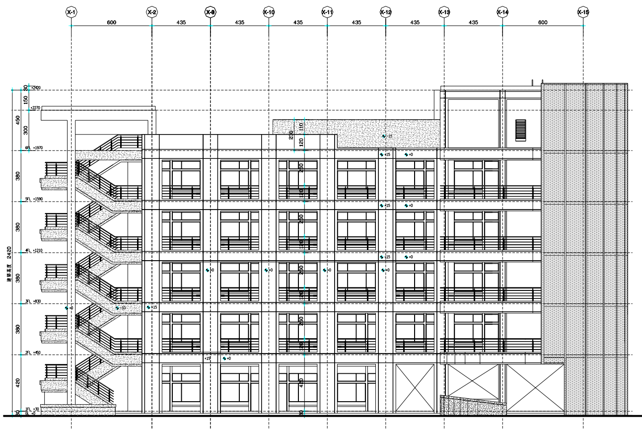
南向立面圖
