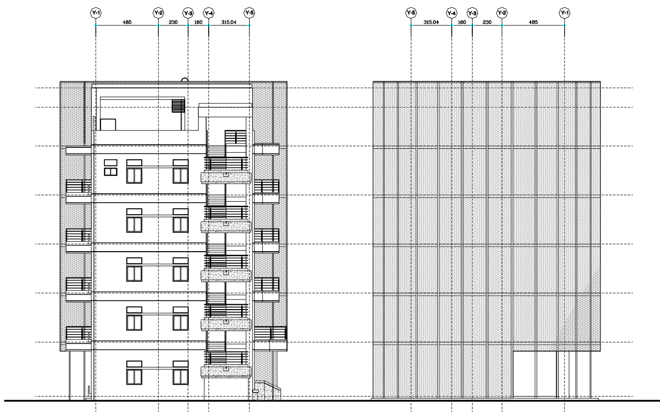
西向立面圖
