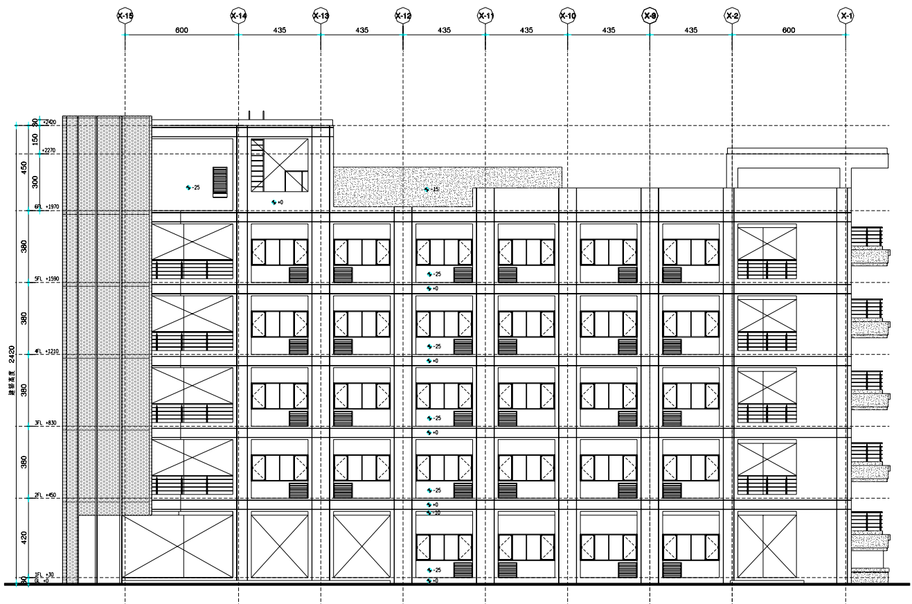
北向立面圖
