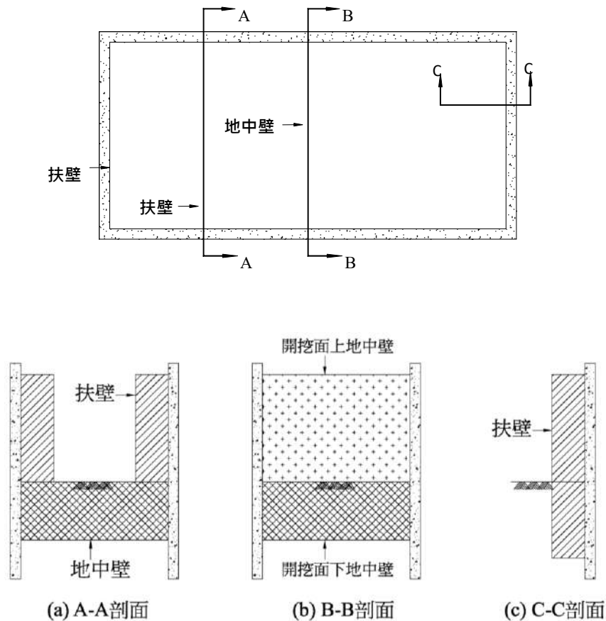
圖-解 8.7-1 地中壁及扶壁示意圖
