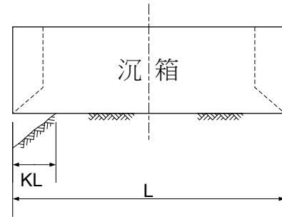
圖-解 6.2-12 懸臂支承狀況
