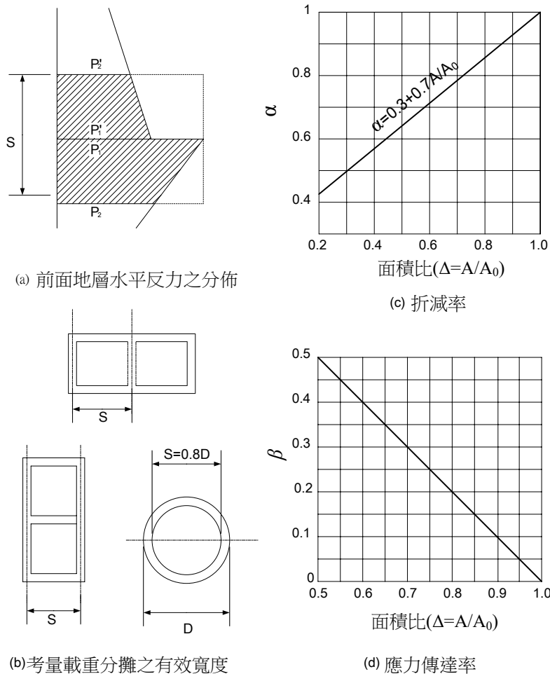
圖-解 6.2-15 完成後之載重狀況
