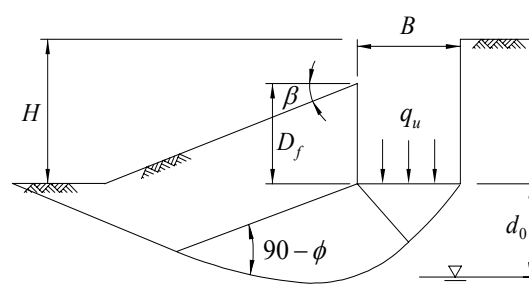
圖-解 4.3-6 坡面上之基礎破壞模式
