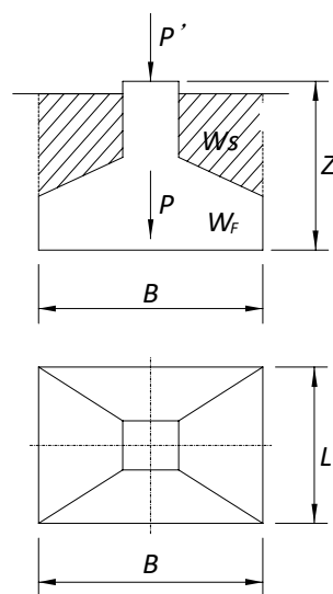
圖-解 4.1-1 獨立基腳載重示意圖
