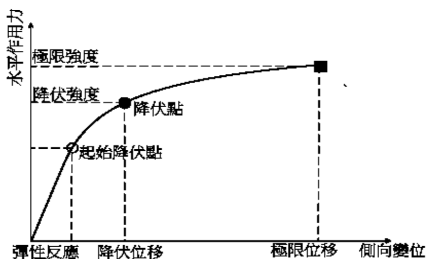
圖-解 5.3-8 基樁側向承載反應曲線示意圖
