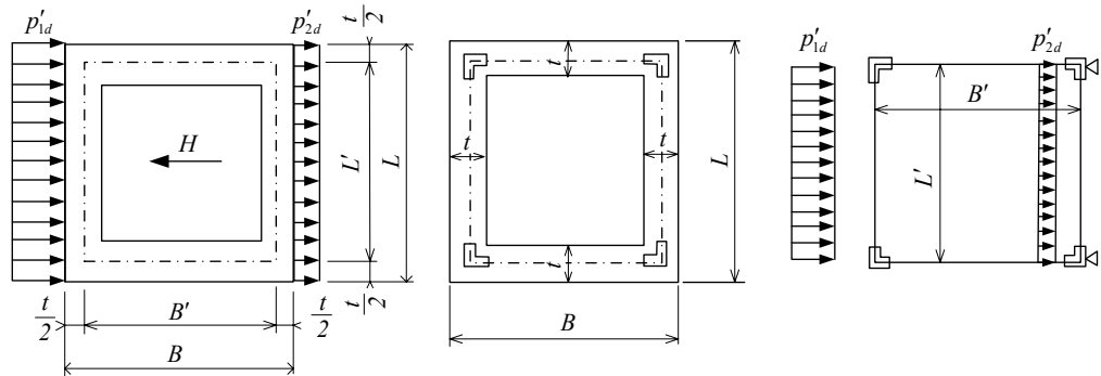
(a)推算剖面力時用的載重
