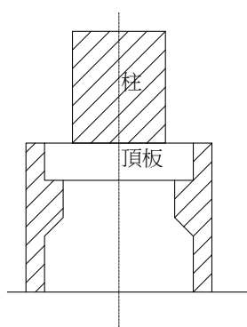
圖-解 6.2-18 沉箱懸吊狀態之設計
