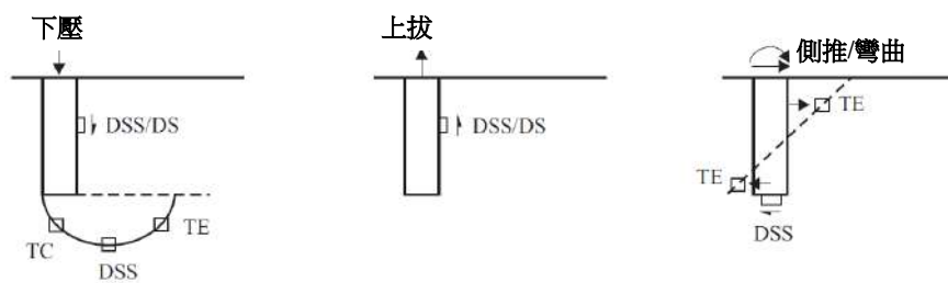
(d) 短樁或沉箱
