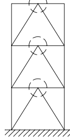
圖C13.8-4 倒V型斜撐構架
