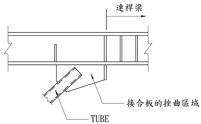
圖C13.9-6 不良之斜撐與連桿梁接合細部
