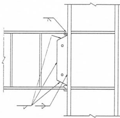
圖C13.9-5 剪力連桿與柱接頭細部
