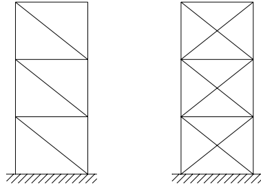
圖C13.8-1 對角型斜撐構架
