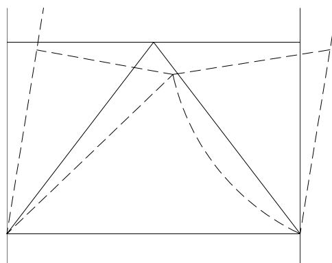
圖 C13.8-8 倒 V 型斜撐構材之破壞機構
