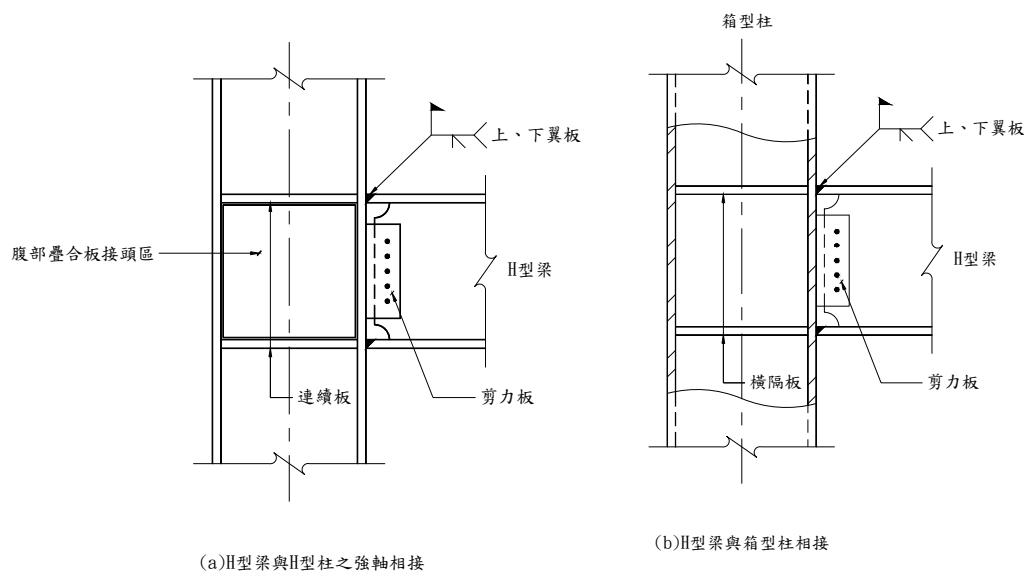
圖C13.6-1 傳統翼板全滲透銲腹板栓接梁柱接頭
