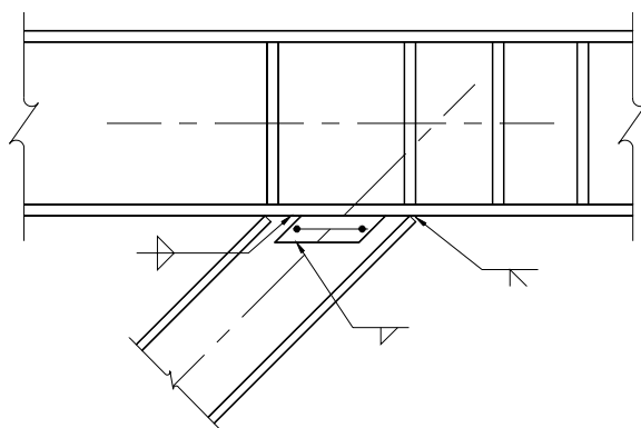
圖C13.9-8 H型斷面斜撐與連桿梁接合細部
