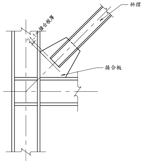
圖 C13.8-7 斜撐構材面外挫屈時接合板之設計
