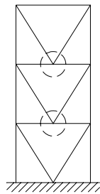
圖C13.8-3 V型斜撐構架
