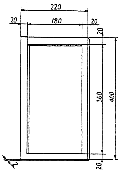
試樣固定框
