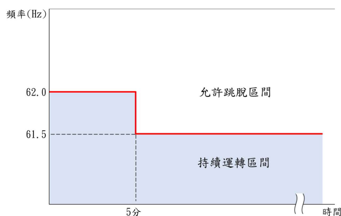
圖 4 高頻率持續運轉能力示意圖
