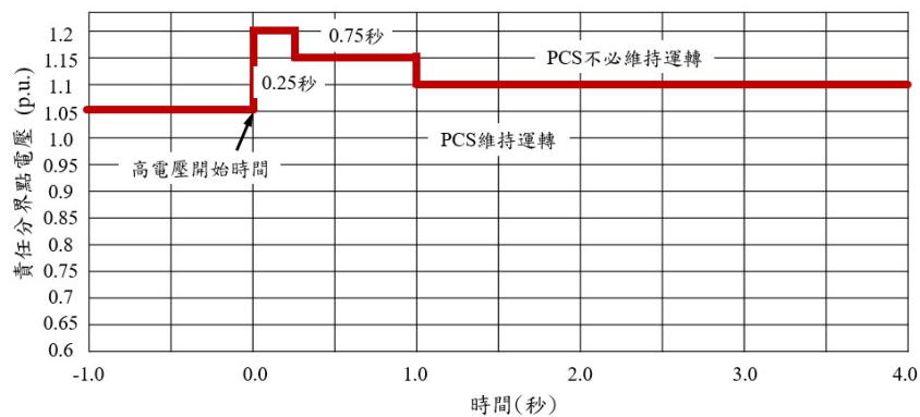
圖 2 高電壓持續運轉能力示意圖
