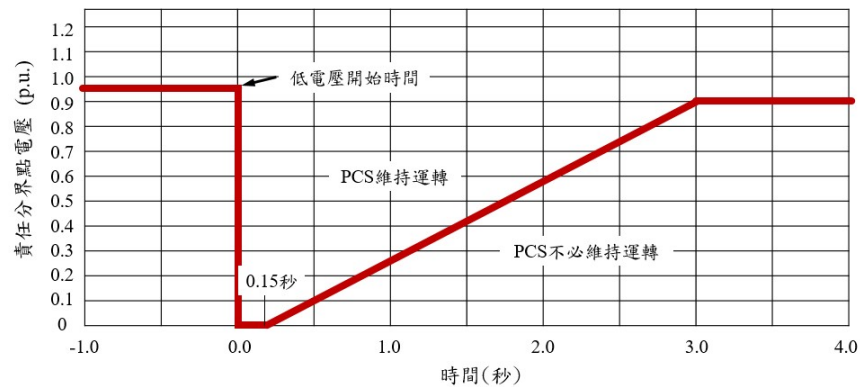
圖 1 低電壓持續運轉能力示意圖
