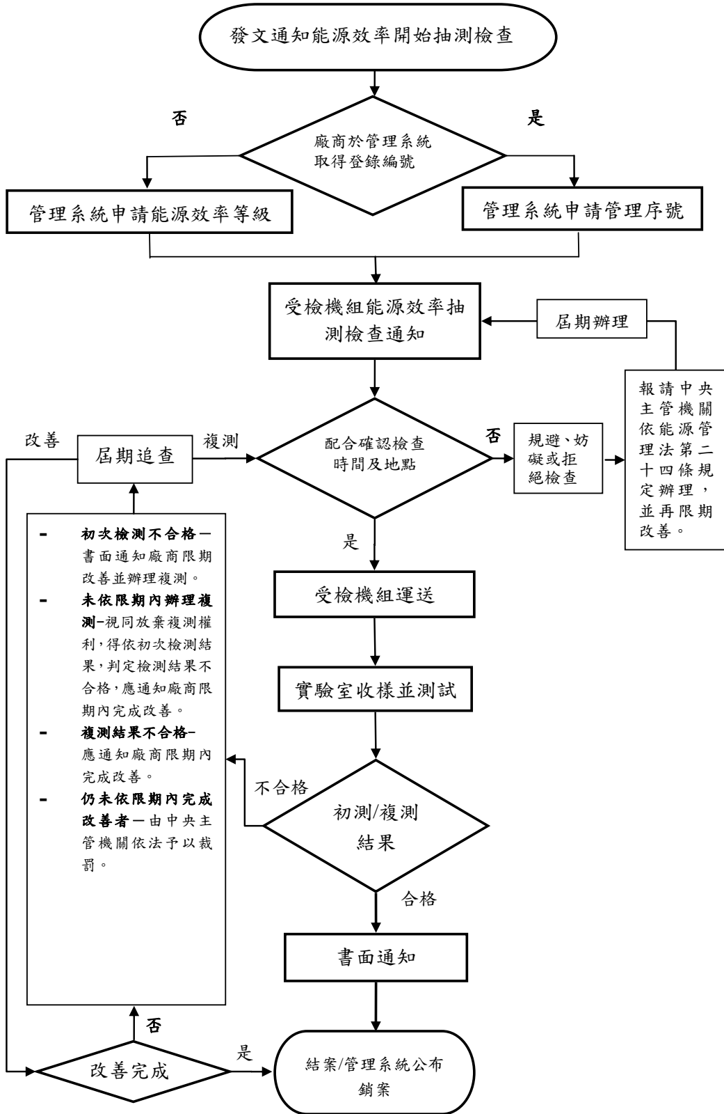
附圖二、能源效率抽測檢查流程圖
