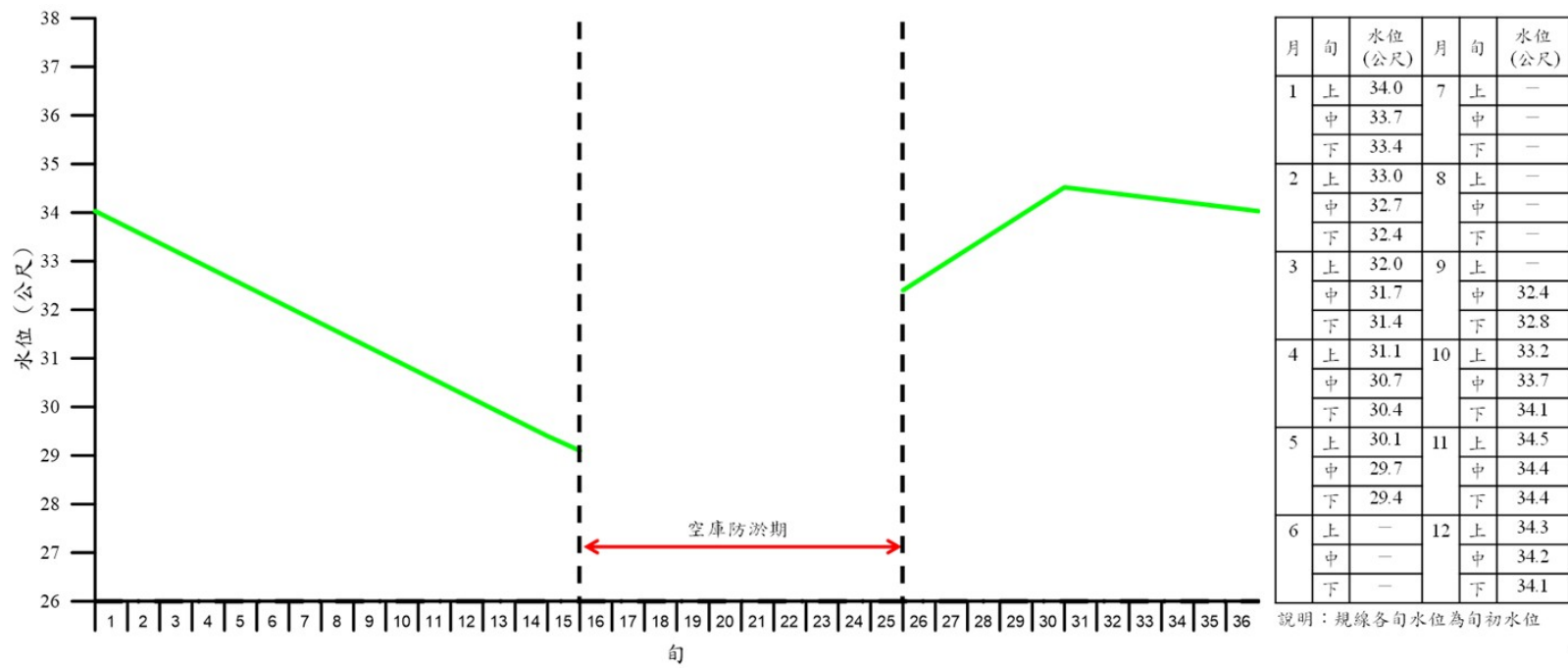
附圖 阿公店水庫運用規線
