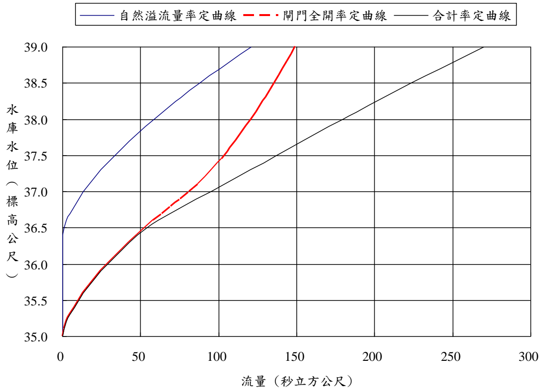
附圖一 自由溢洪道水庫水位與溢流量關係曲線
