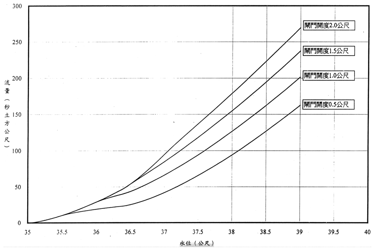
附圖二 溢洪道閘門開度與流量關係曲線
