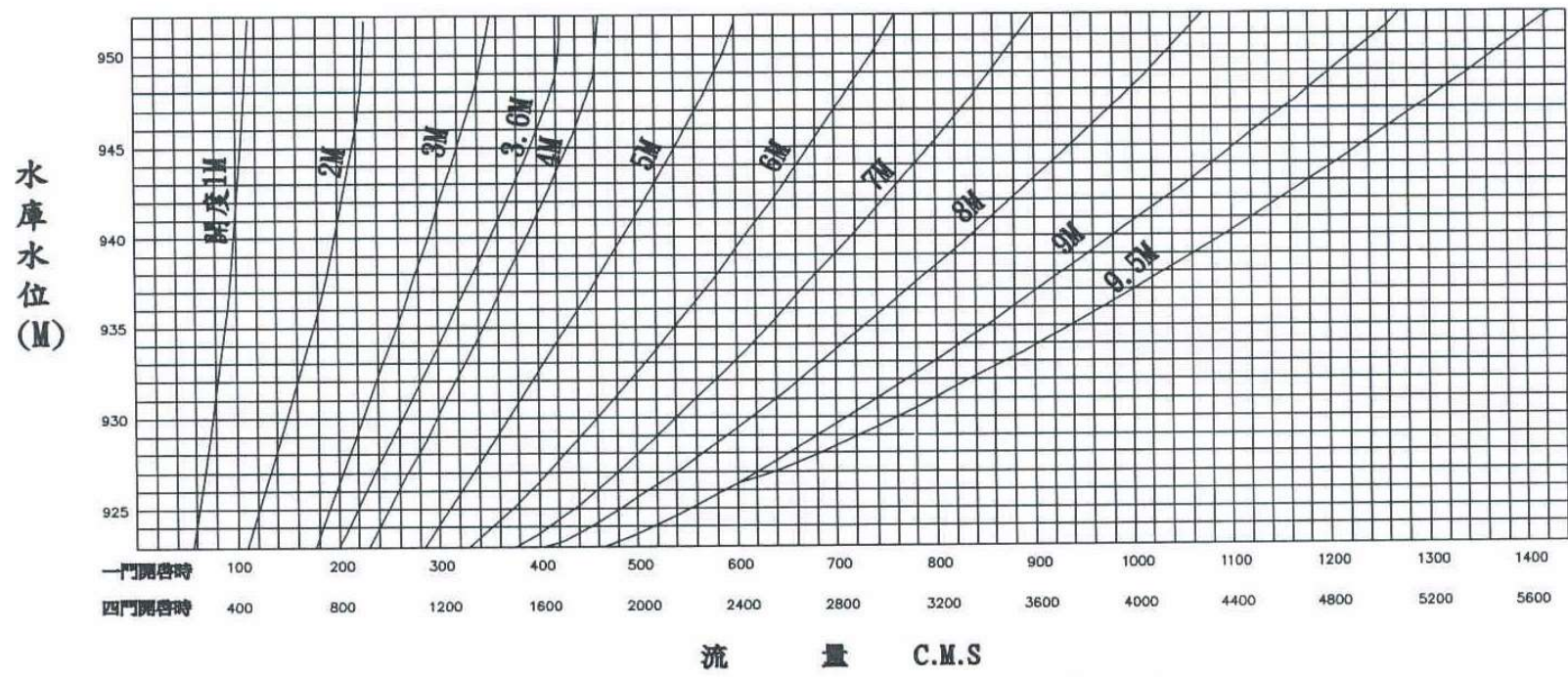
附圖一 谷關水庫壩身排洪閘門率定曲線
