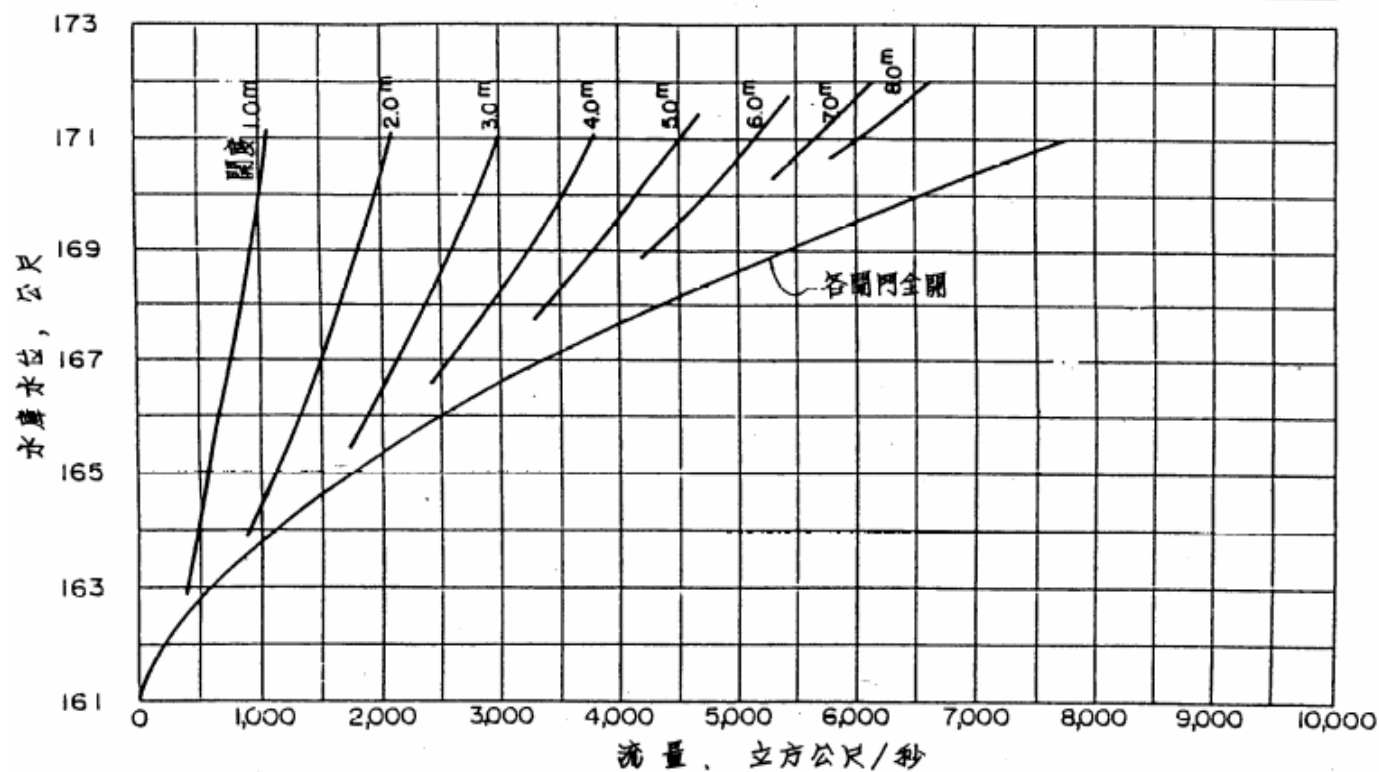
附圖一、溢洪道流量與閘門開度及水庫水位關係曲線
