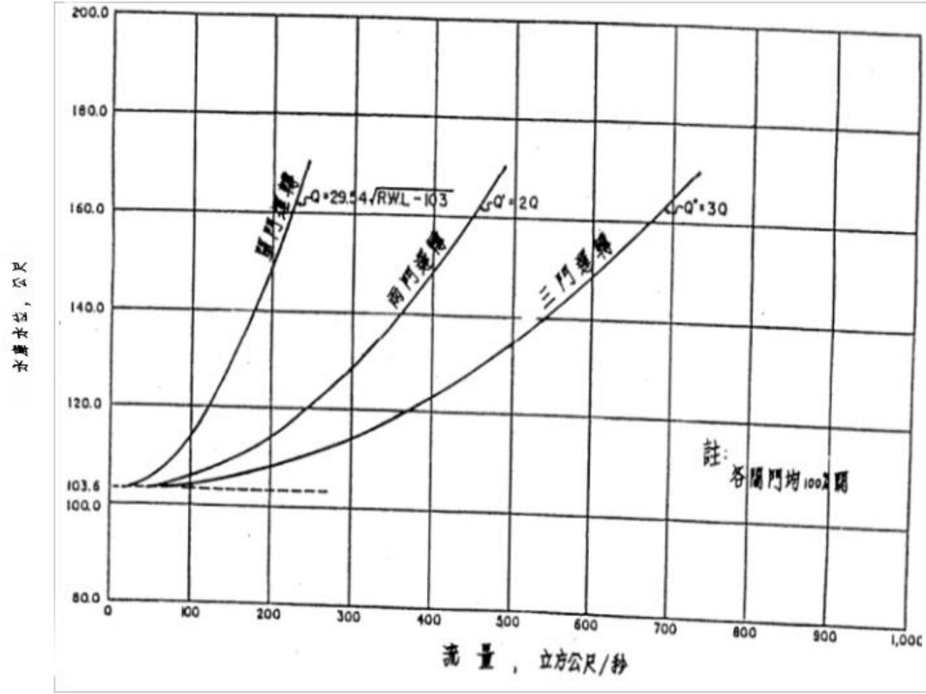
附圖二、沖刷道流量與水庫水位關係曲線
