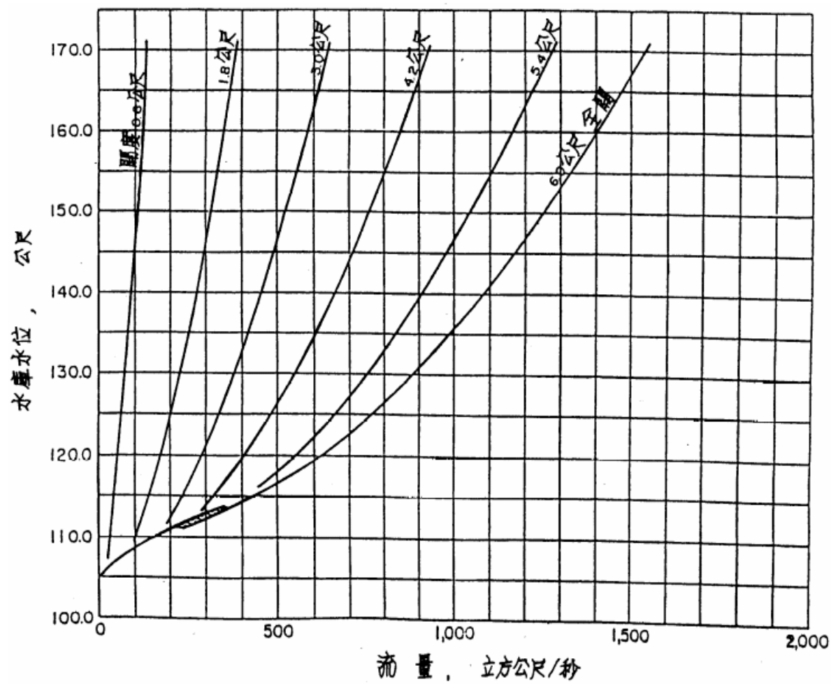
附圖三、排洪隧道流量與閘門開度及水庫水位關係曲線
