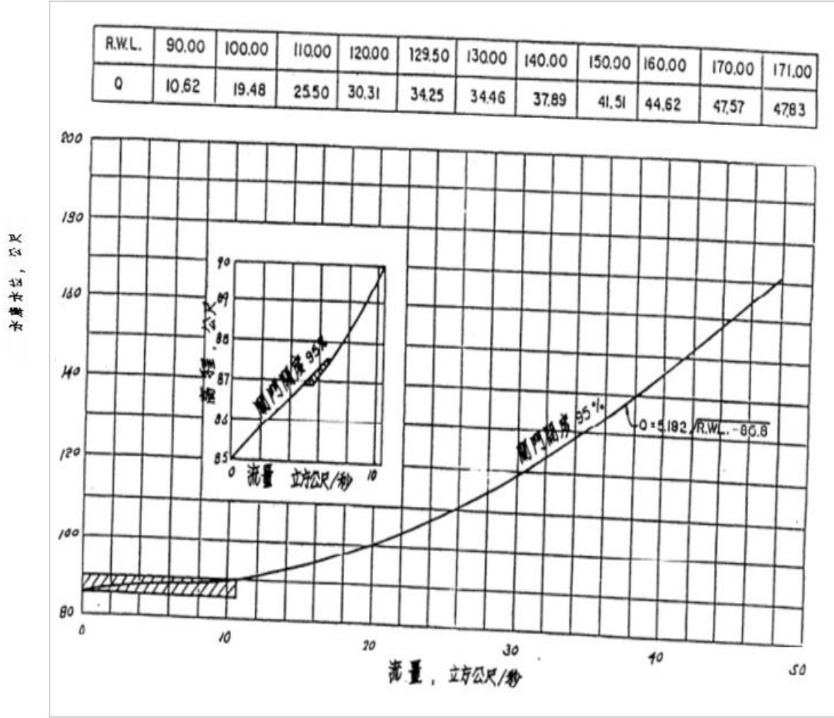
附圖四、河道放水口流量與水庫水位關係曲線
