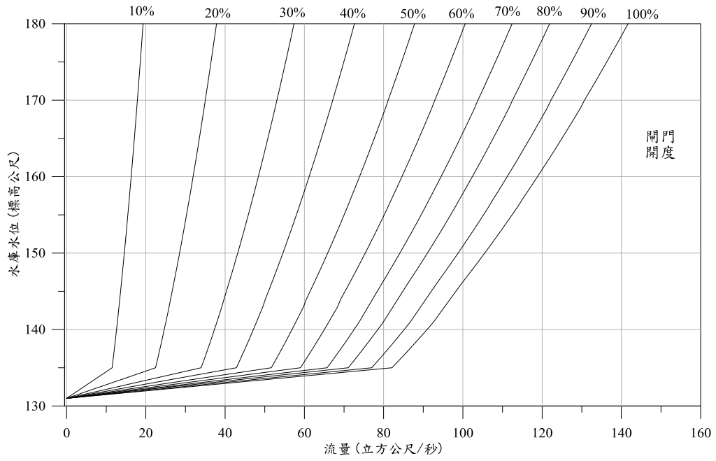
排水道流量率定曲線(控制閘門)
