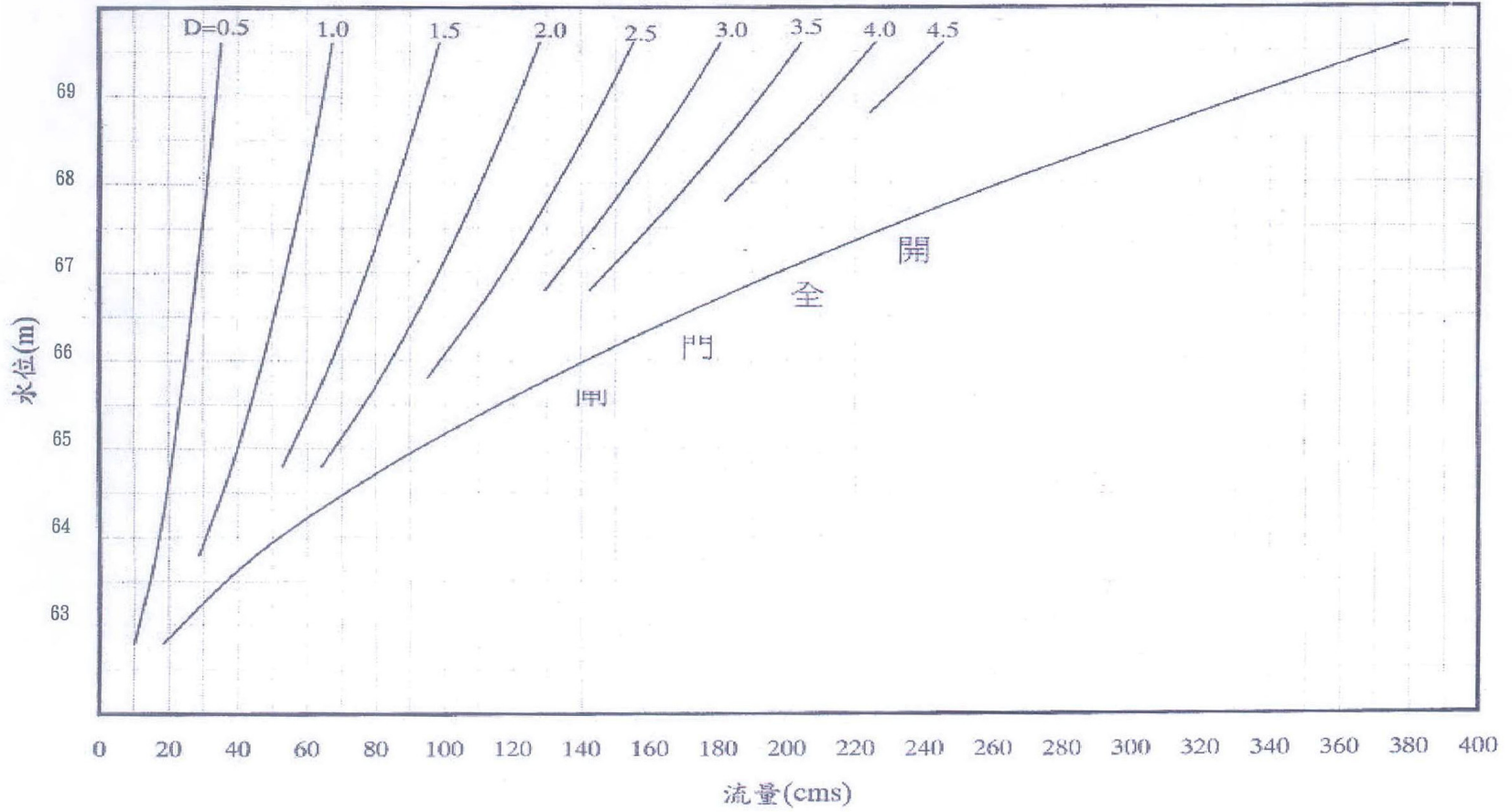
大埔水庫溢洪道流量率定曲線（單座閘門）
