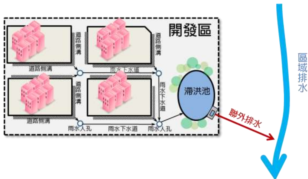
附圖 3 開發基地聯外排水示意圖
