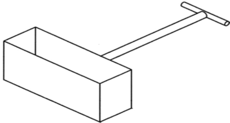
圖一 下墜式採樣箱
