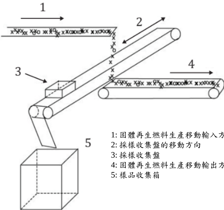
圖四 下墜式物料採樣設備
