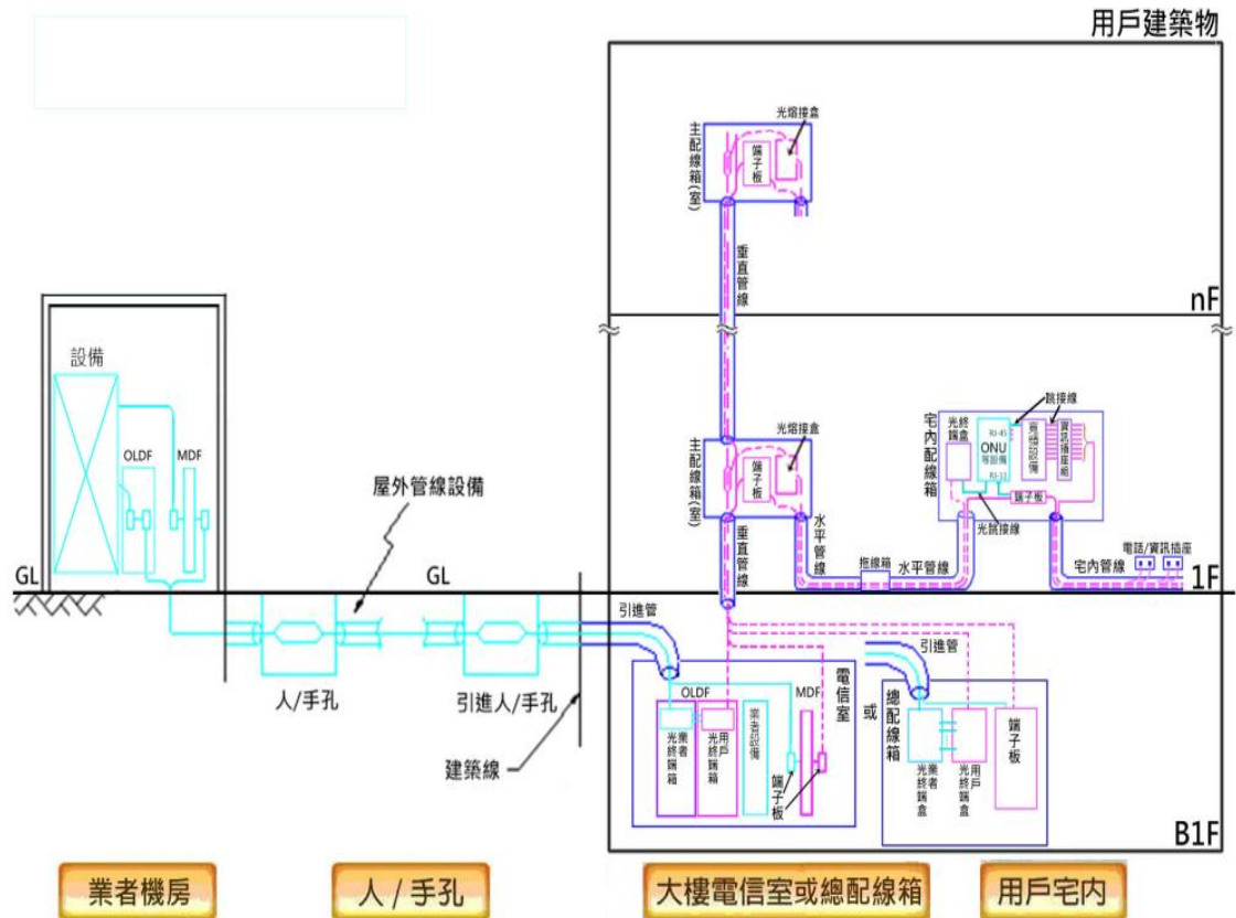
圖4-1 建築物屋內外電信設備示意圖
