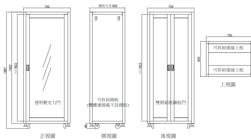
圖6-5 19" 41U加寬型機櫃圖
