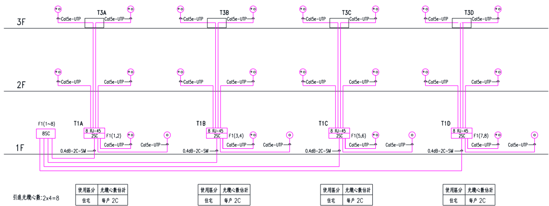
圖17-6 設計範例(二) 光纜及資訊纜線昇位圖
