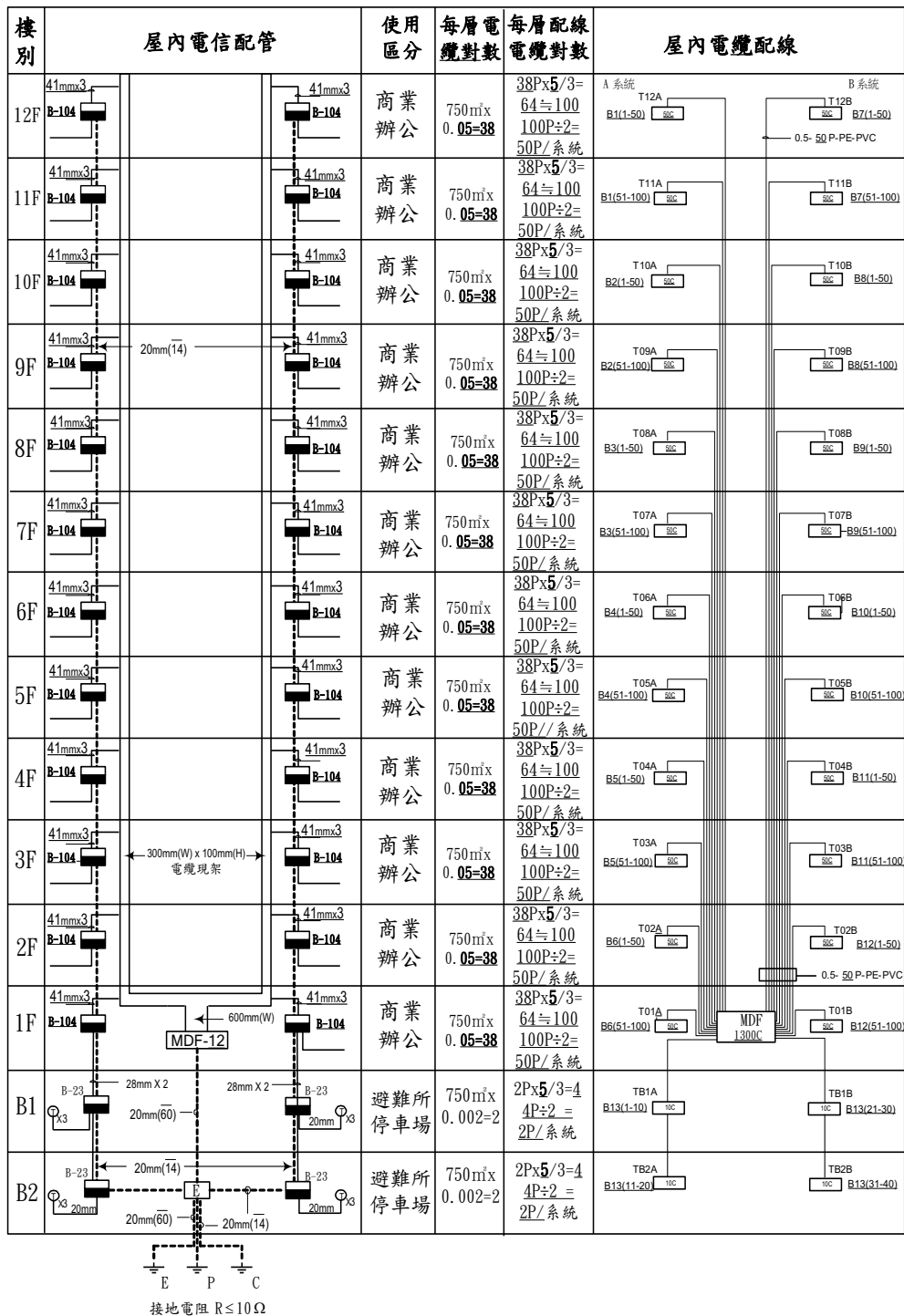
圖 7-3 十二樓舍地下室電信配管線垂直昇位
