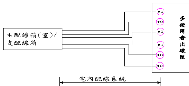
圖4-10 多使用者出線匣配線系統架構圖
