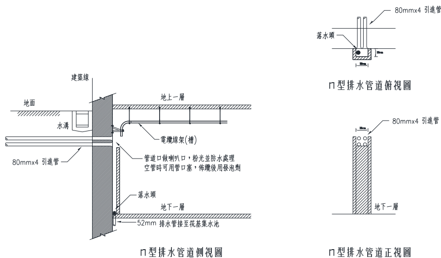
圖15-1 ㄇ型排水管道配置圖
