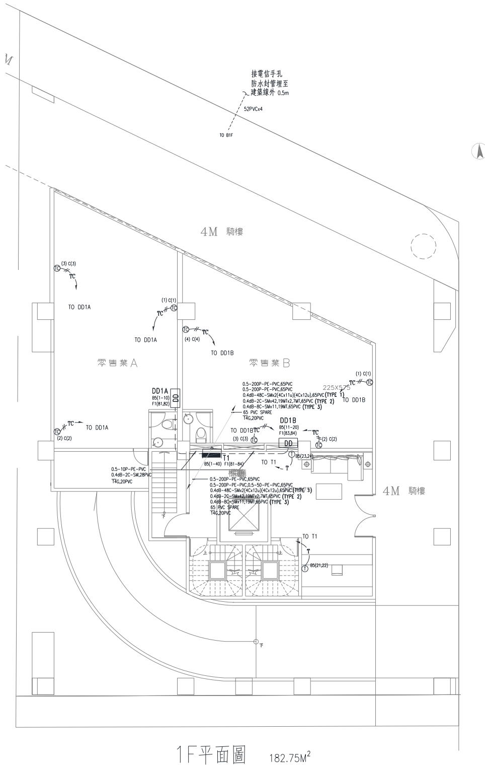
圖7-12 集合住宅一層電信平面圖
