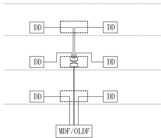
圖4-8 主幹配線中間交接架構圖
