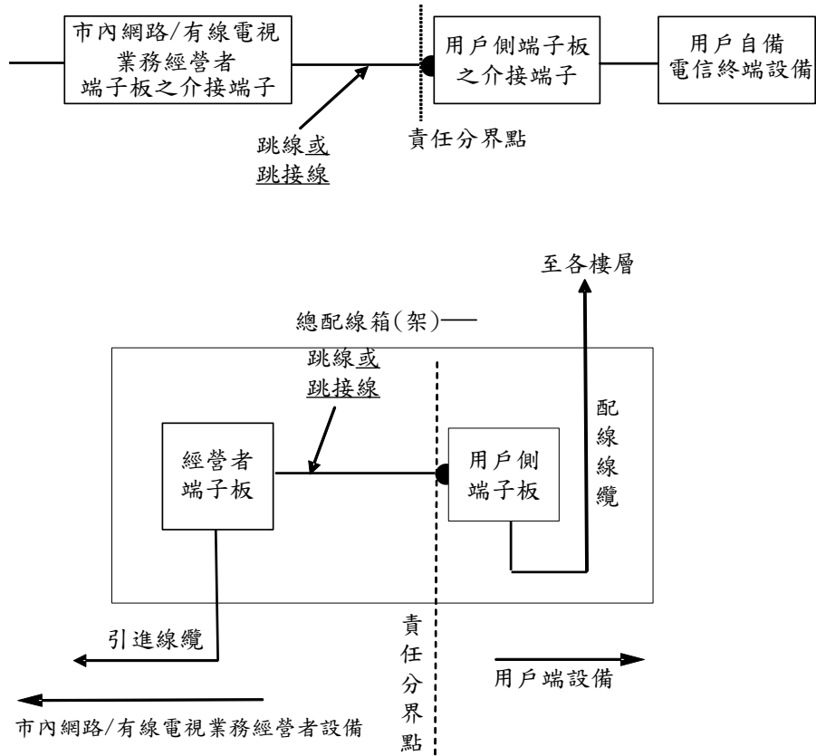
圖5-1 建築物設置用戶側端子板設備者之責任分界圖
