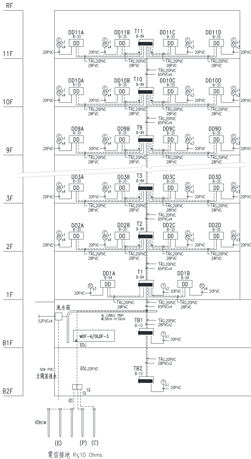
圖7-4 電信配管昇位圖
