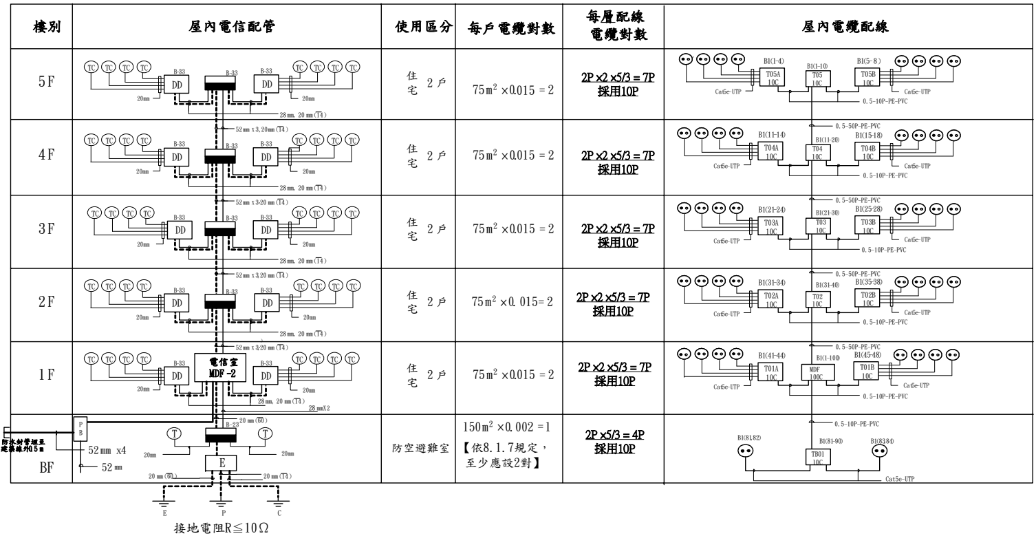
圖 7-2 五樓電信管線垂直昇位圖
