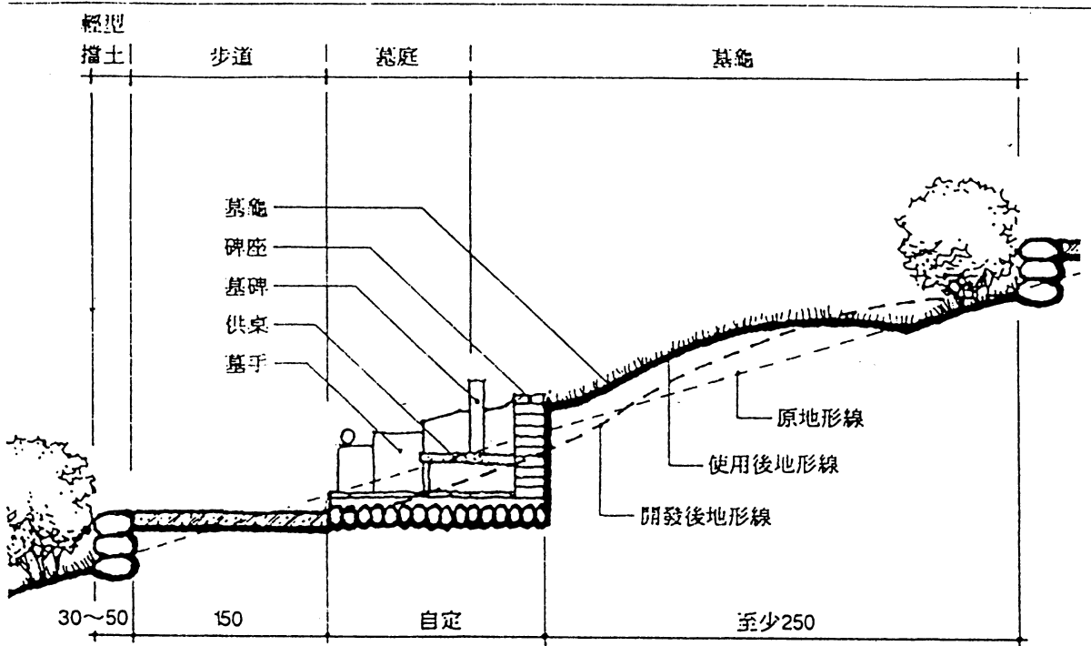
圖1 墓區開發細部範例 - 剖面開發型態
