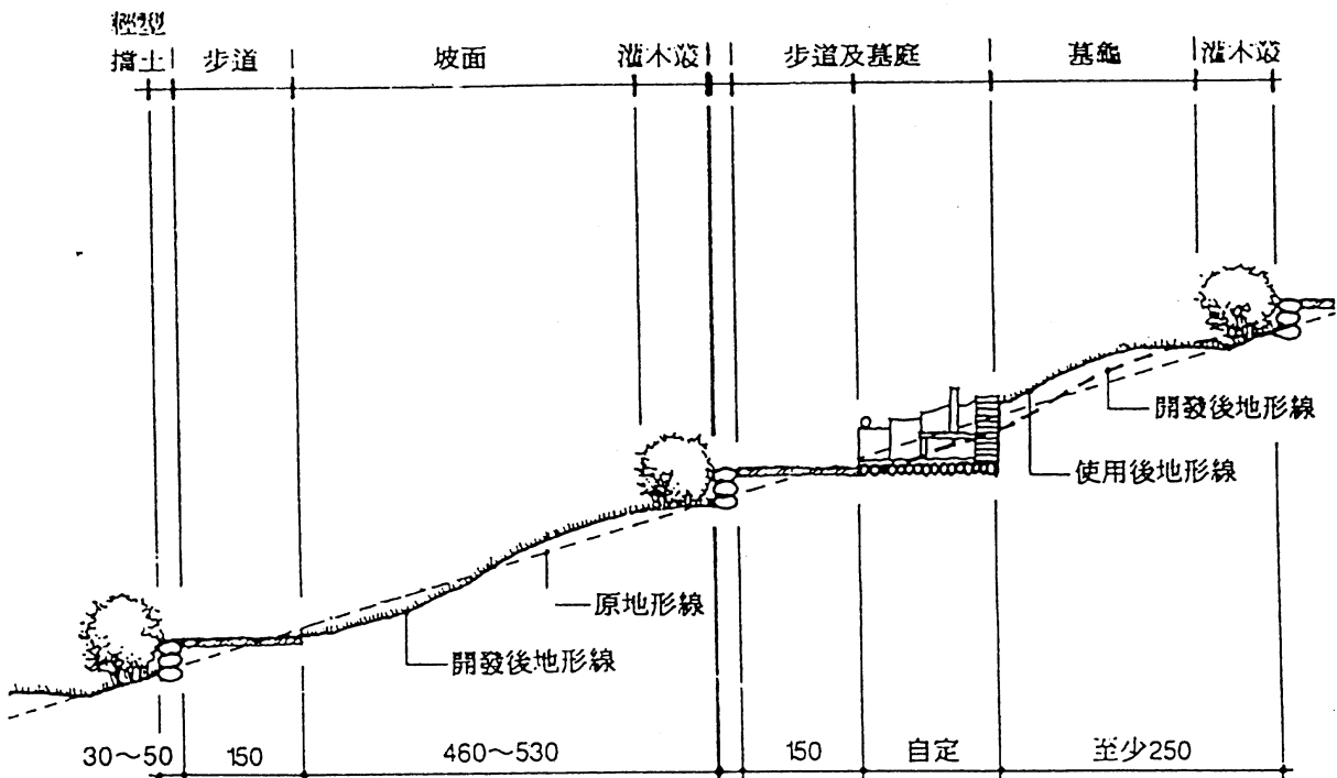
圖3 墓區開發細部範例 - 坡度30%之開發剖面示意
