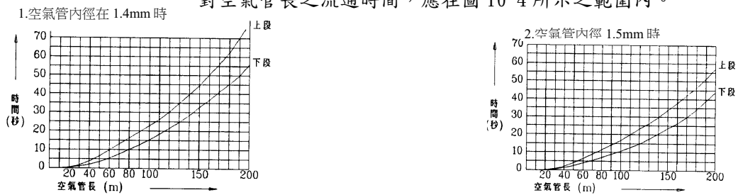
圖 10-4 空氣管流通曲線
