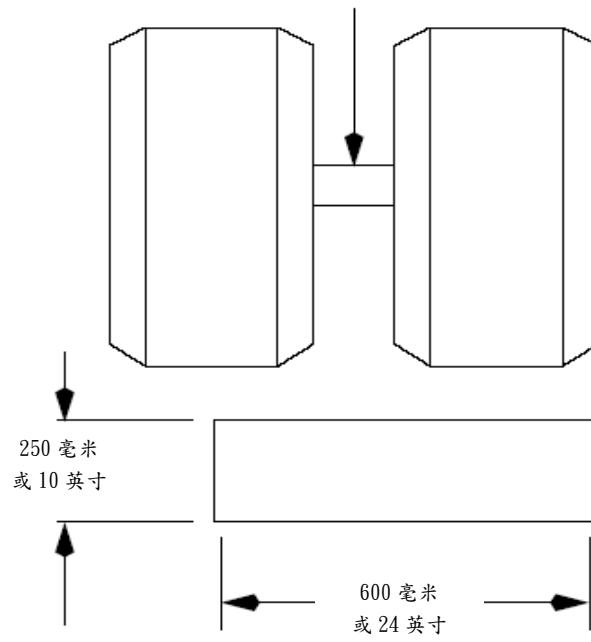
圖二二六～二 車輪荷重面積
