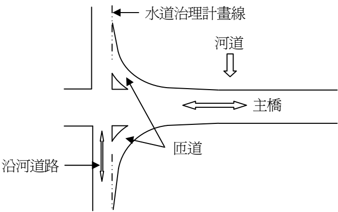
直接式匝道示意圖
