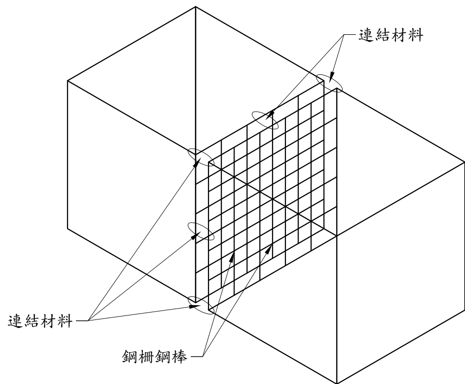
鋼柵石籠籠體連結示意圖
