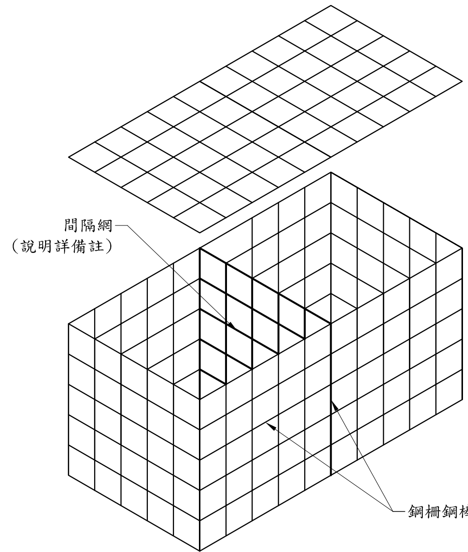
鋼柵石籠長度2m以上籠體組合示意圖
