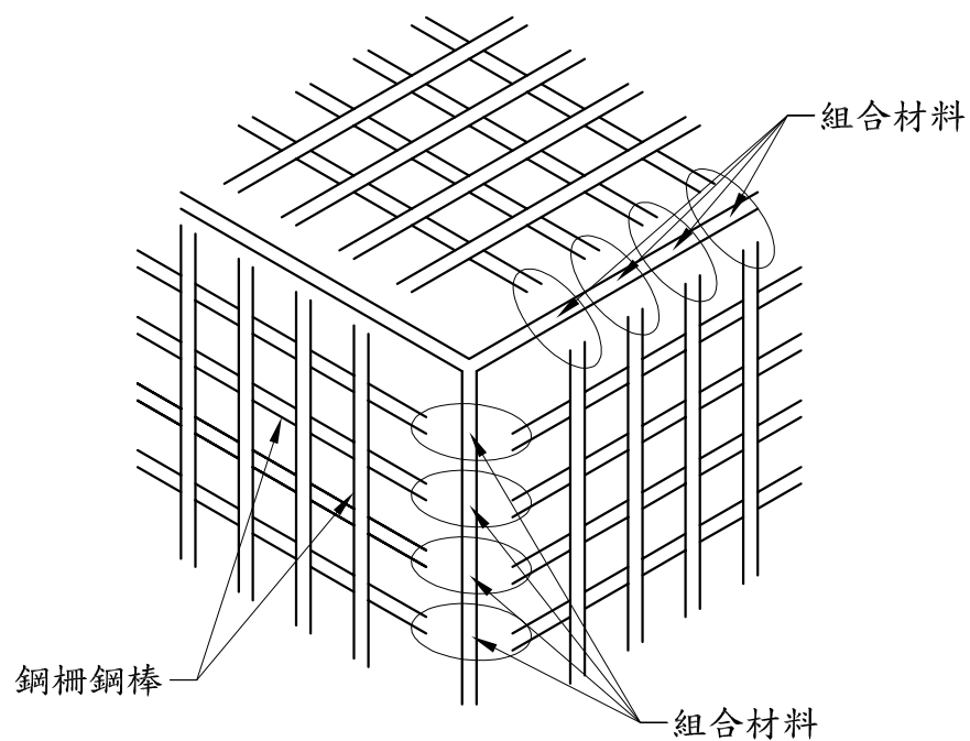
鋼柵石籠籠體組合示意圖
