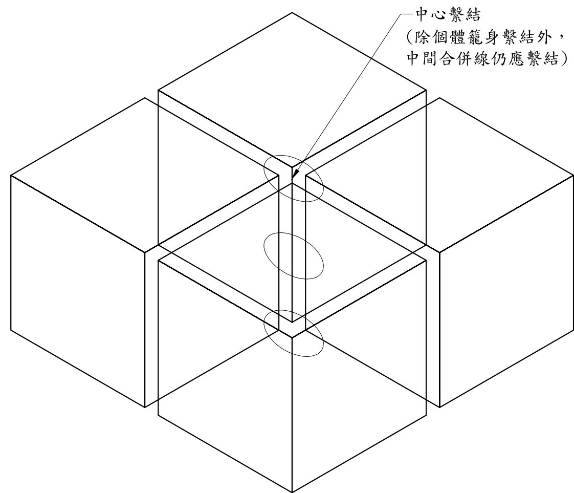
鋼柵石籠四籠合併籠體示意圖
