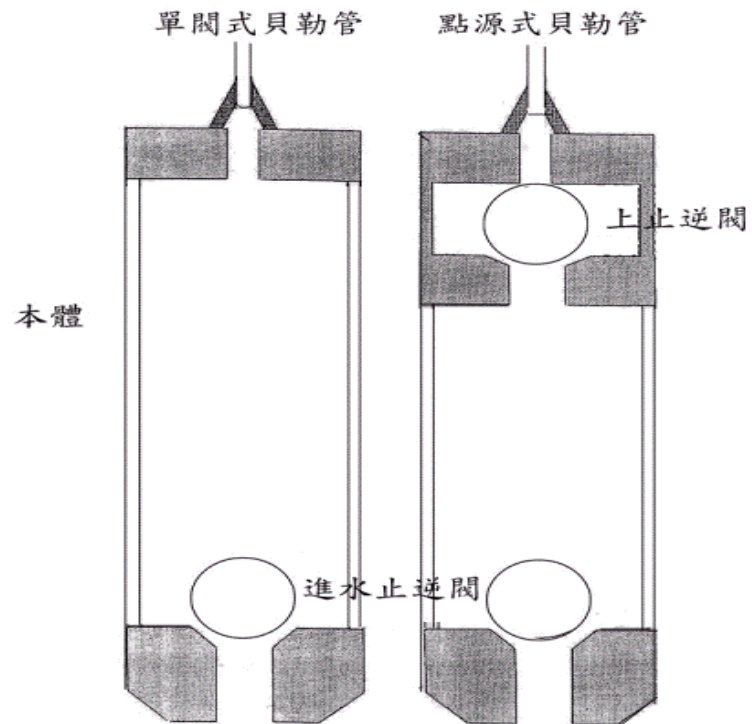
圖二 貝勒管構造示意圖
