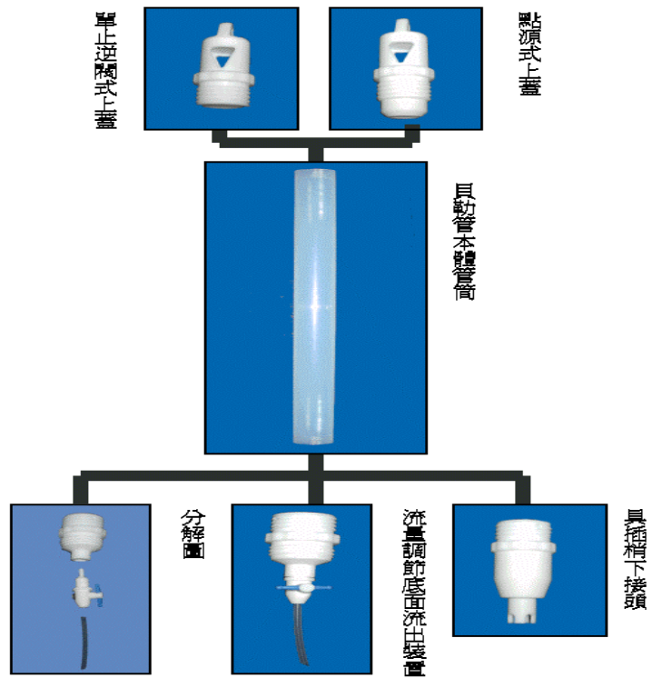
圖一 貝勒管及其配件
