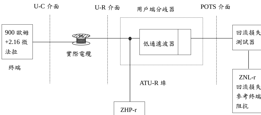
圖八 回流損失測試接線圖
