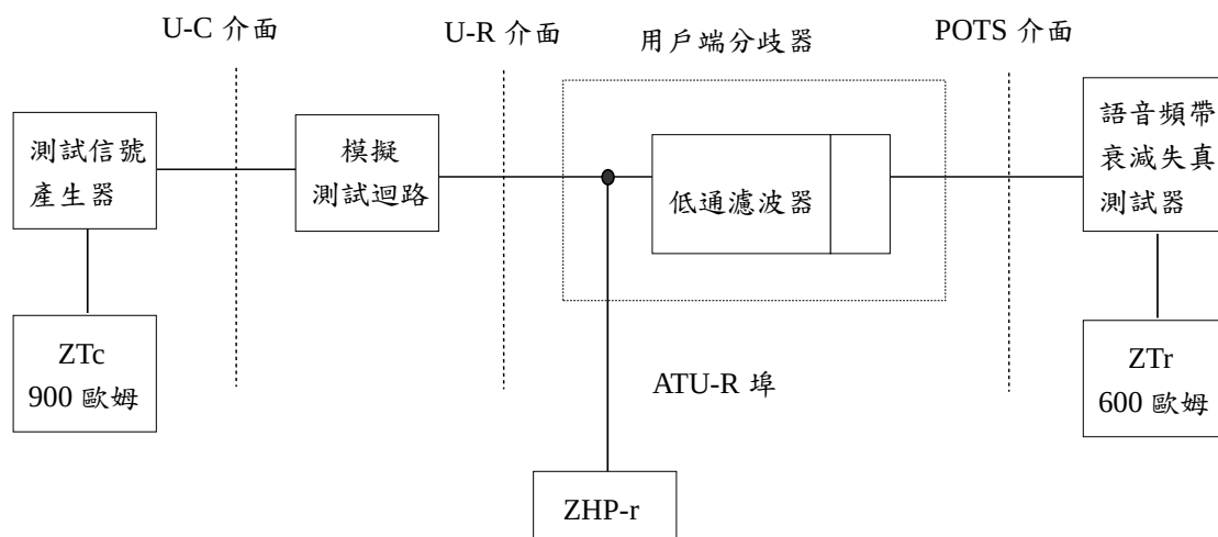
圖六 語音頻帶衰減失真測試接線圖
