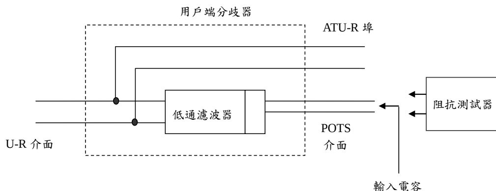
圖十 用戶迴路負載電容測試接線圖
