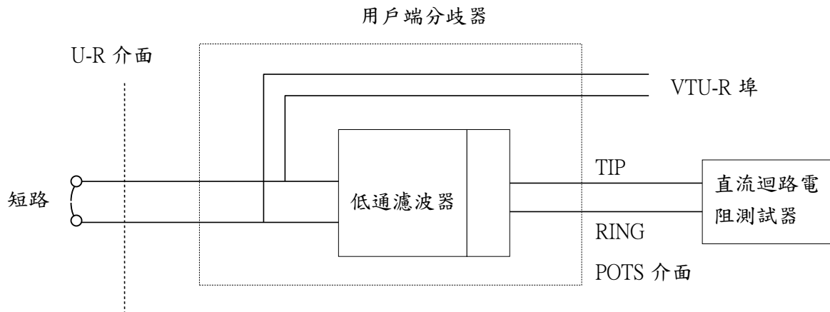
圖一 POTS 介面上 TIP 至 RING 的直流電阻測試
