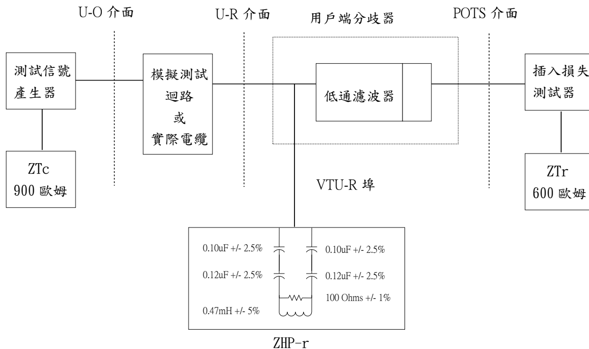
圖三 語音頻帶插入損失測試接線圖
