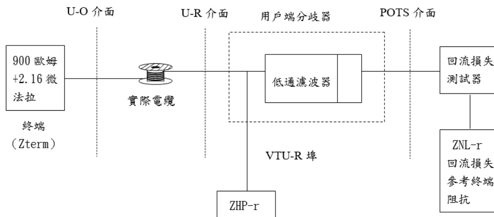
圖八 回流損失測試接線圖
