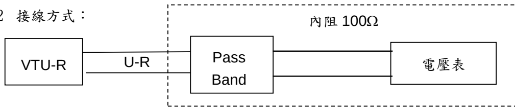
圖十三 VTU-R 發送信號總功率測試架構圖
