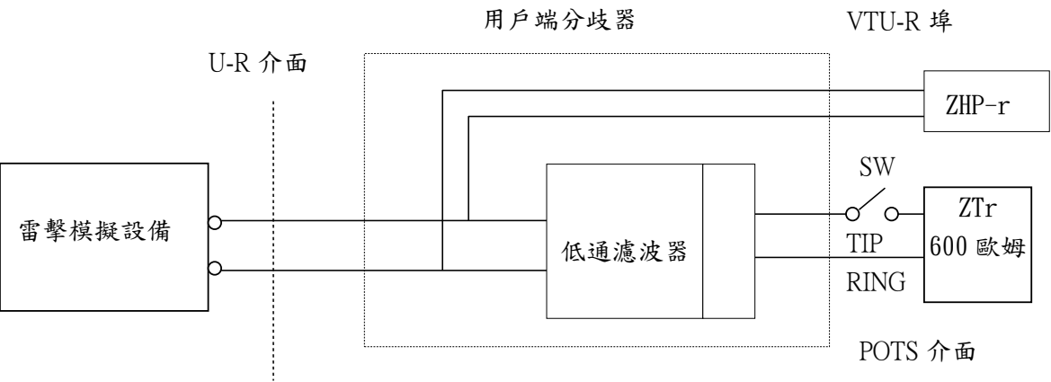
圖十一 雷擊試驗接線圖
