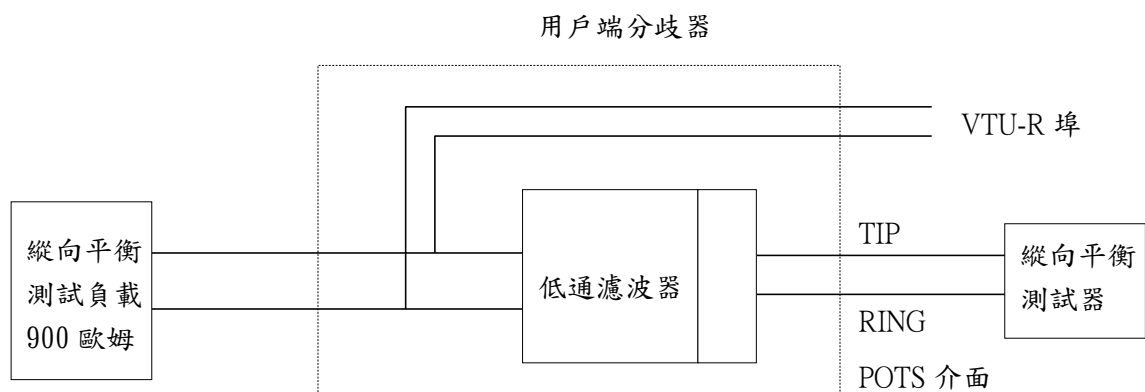
圖九 縱向平衡測試接線圖
