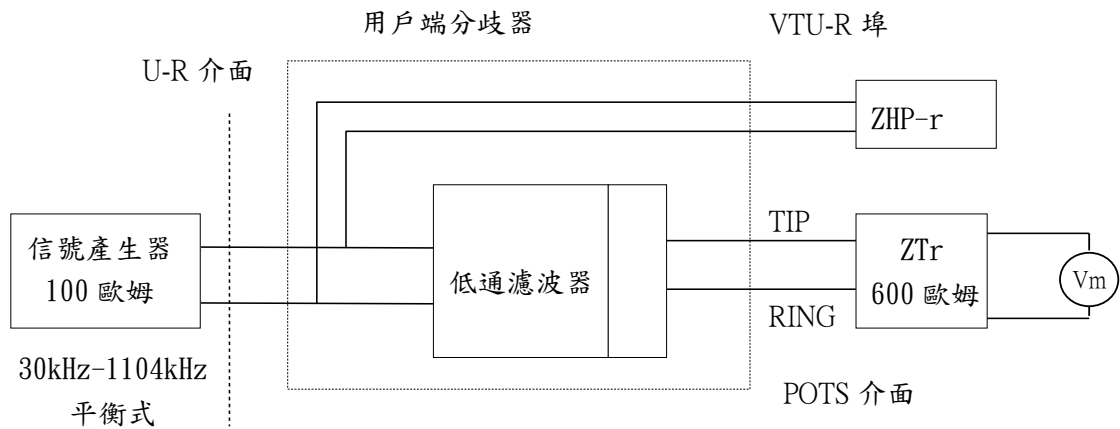
圖四 30kHz-1104kHz 頻帶信號衰減測試接線圖
