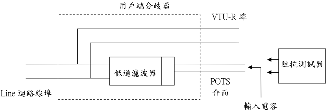
圖十 用戶迴路負載電容測試接線圖
