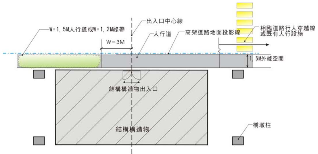
附圖五: 構造物出入口位於車道側時， 人行道留設方式示意圖
