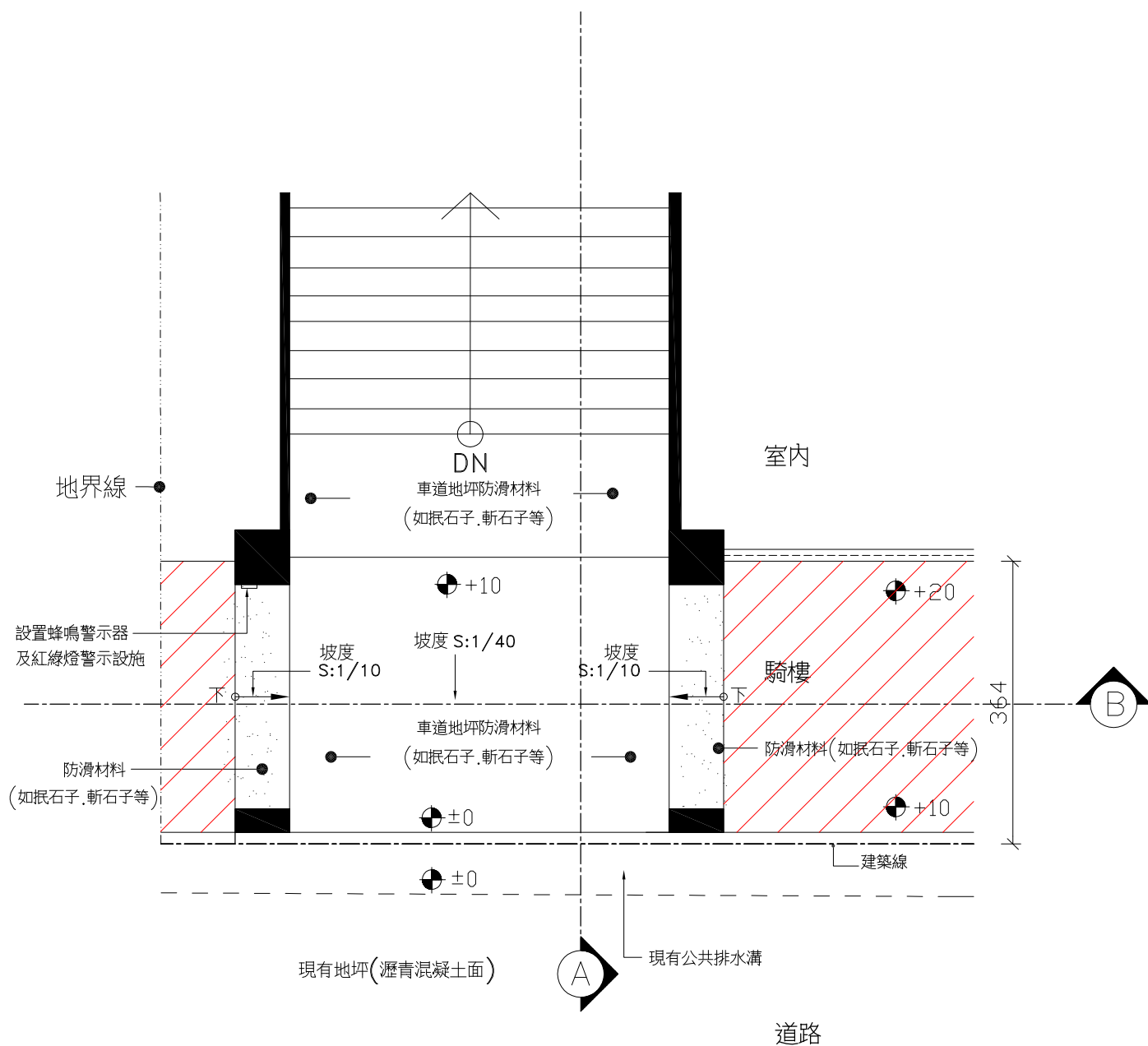
車道出入口平面圖
